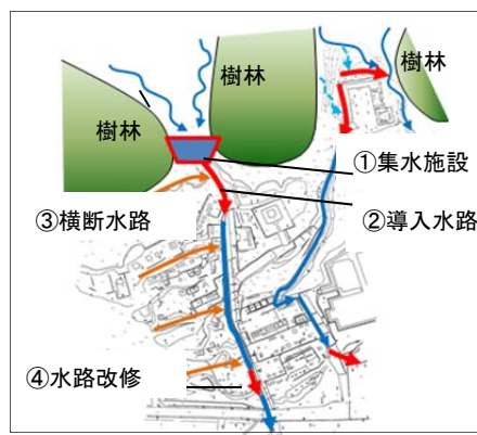
集水施設と導入水路
