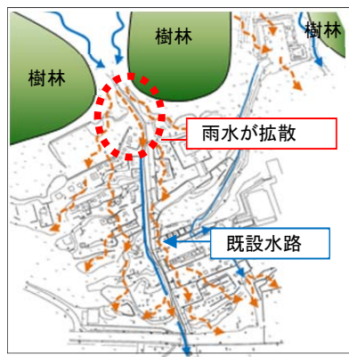
自然水路で雨水拡散
